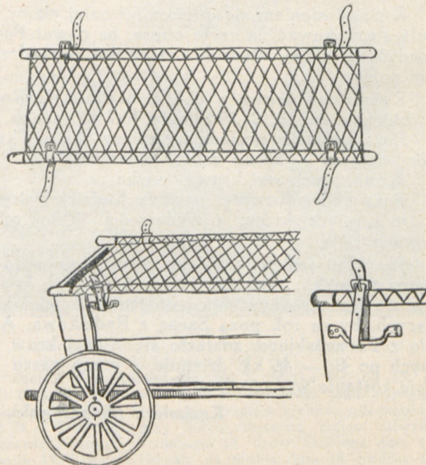
Siatka na wóz do przewożenia świń.
