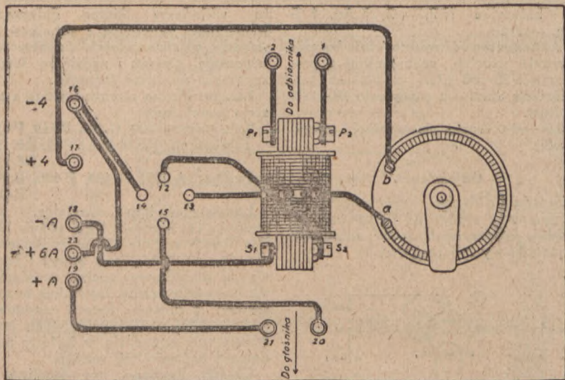
Schemat montażowy.
