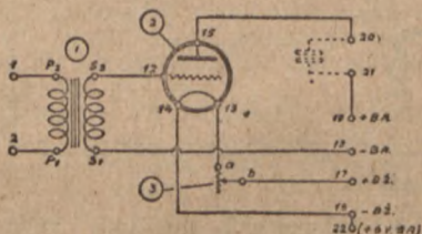
Schemat teoretyczny.
