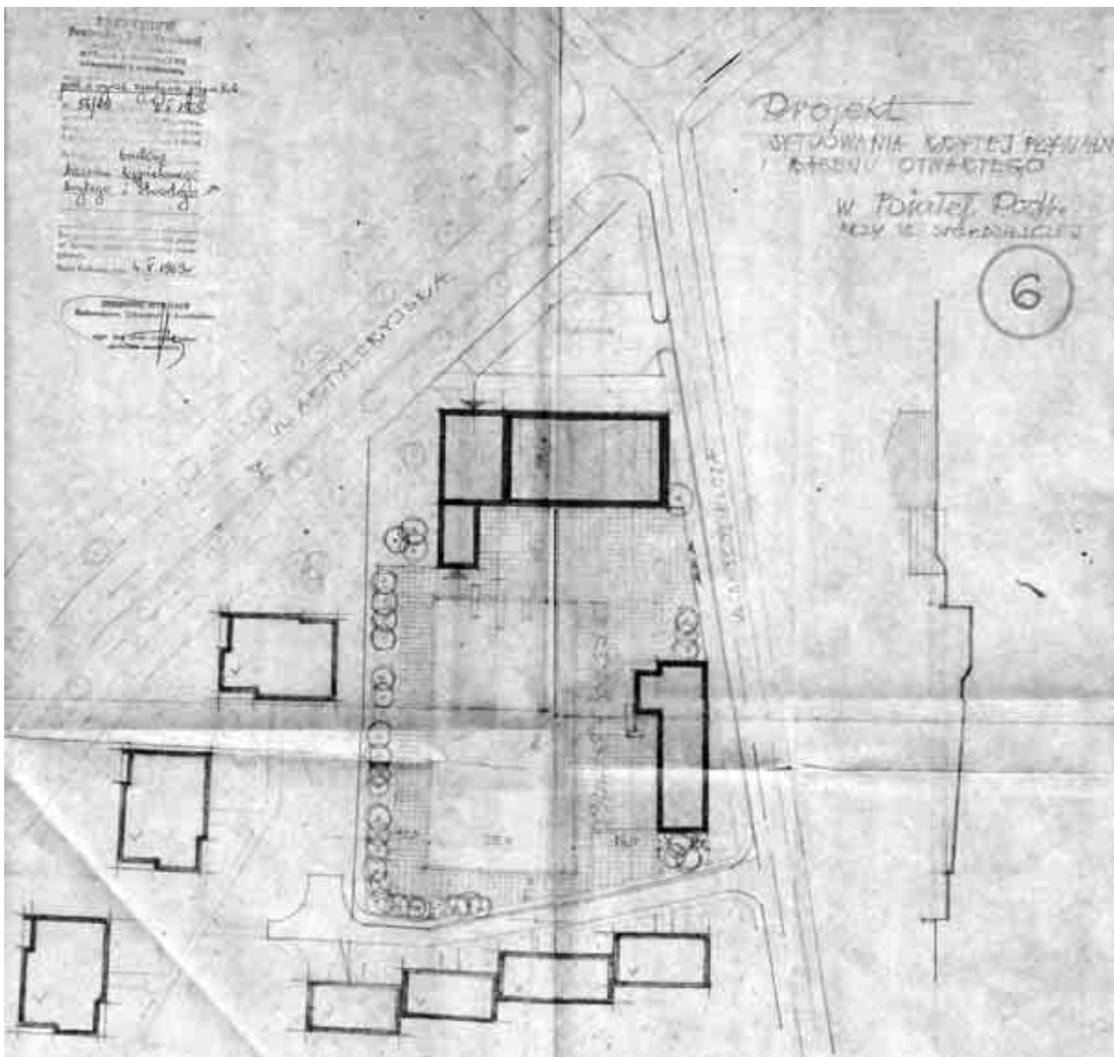
Projekt usytuowania krytej pływalni i basenu otwartego w Białej Podlaskiej przy ul. Spółdzielczej
