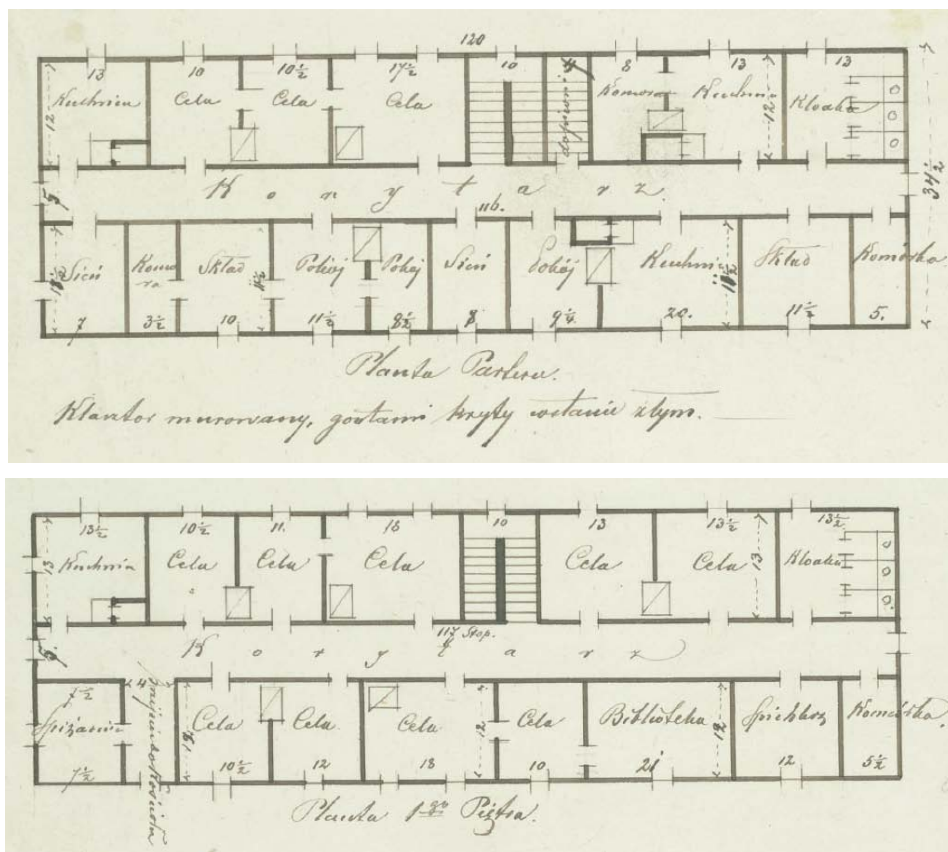
Ryc. 2. Plan parteru i pierwszego piętra klasztoru bazylińskiego w Zamościu w 1865 r. Źródło: AGAD, Zbiory kartograficzne, sygn. teka 21 plan 24, ark.1.
