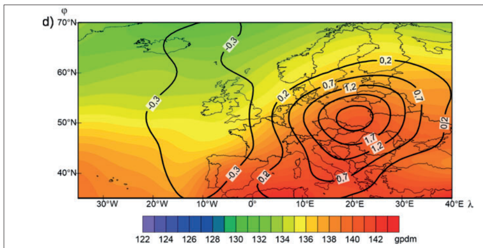
Ryc. 7a–d. Średnia temperatura powietrza ( ^{\circ}\text{C} ) na powierzchni izobarycznej 850 hPa (a i c) i średnia grubość warstwy powietrza 850–1000 hPa (b i d) wraz z odchyleniami od normy (linia) podczas występowania powietrza zwrotnikowego nad Lubelszczyznę wiosną (a i b) i latem (c i d)
