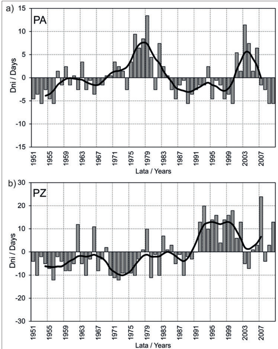
Ryc. 2. Odchylenia rocznej liczby dni z masą powietrza arktycznego (a) i zwrotnikowego (b). Okres referencyjny: 1951–2010
