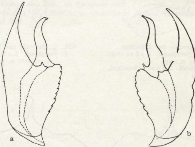
Abb. 6. Sagitta
