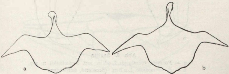
Abb. 4. Subgenitalplatte
