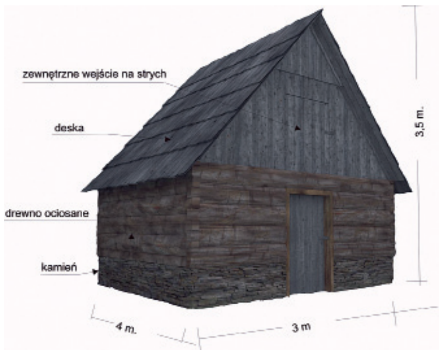
Ryc. 4. Schemat konstrukcyjno-architektoniczny szopy drewniano-kamiennej Fig. 4. Construction scheme of architecture of a wooden-stone shed
