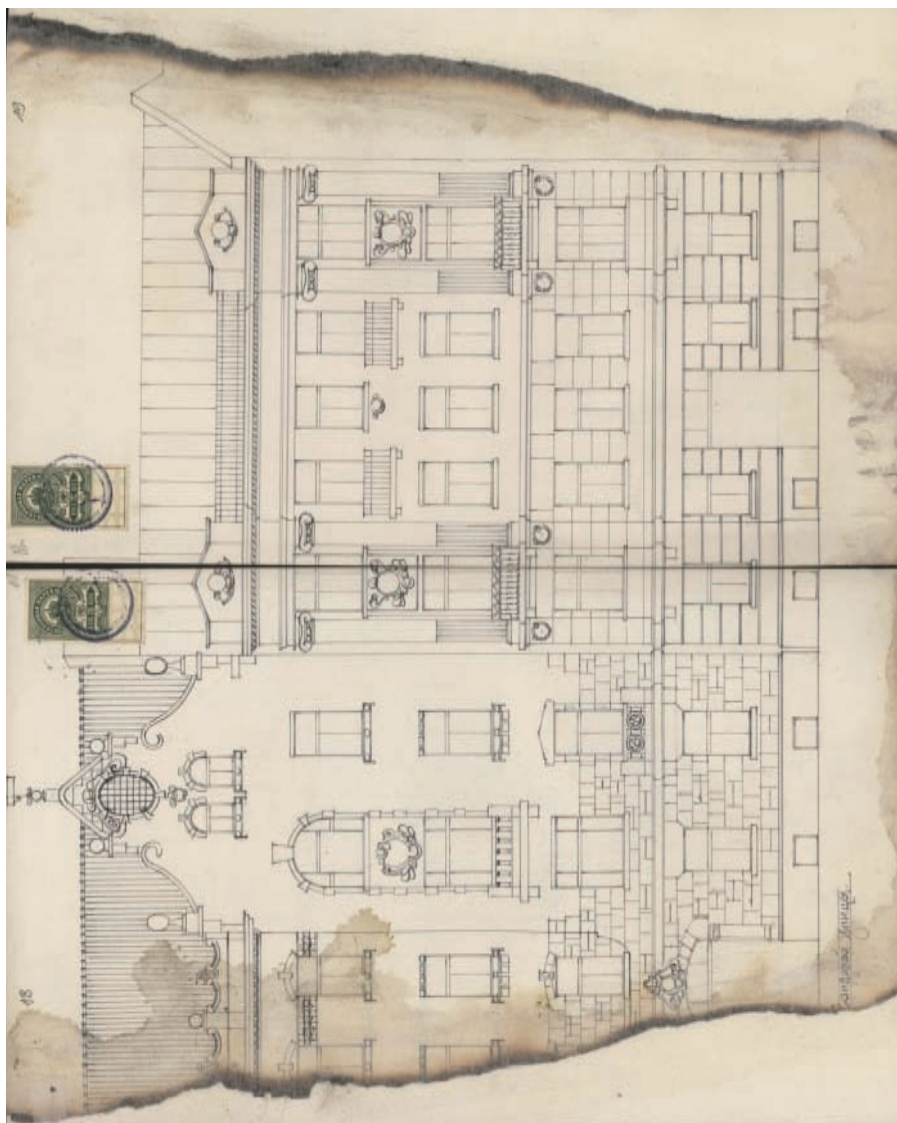
Ilustracja 5. Fragment projektu elewacji frontowej kamienicy przy ul. Chopina 11. APL, RGL (1867–1918), BI, 1912–86, s. 19.
